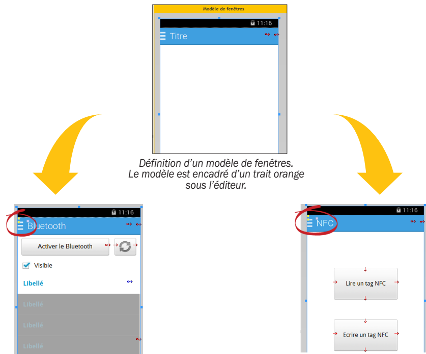
Utilisation du modèle dans plusieurs fenêtres. Les éléments appartenant au modèle sont identifiés par un carré jaune.
